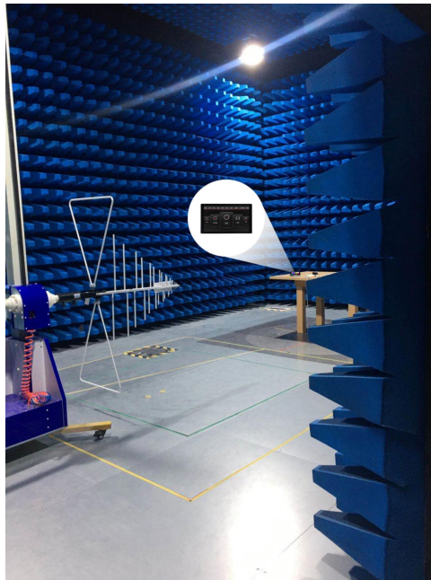
图 4-4 RE 测试图
