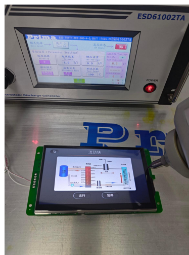
图 4-2 ESD 测试图
